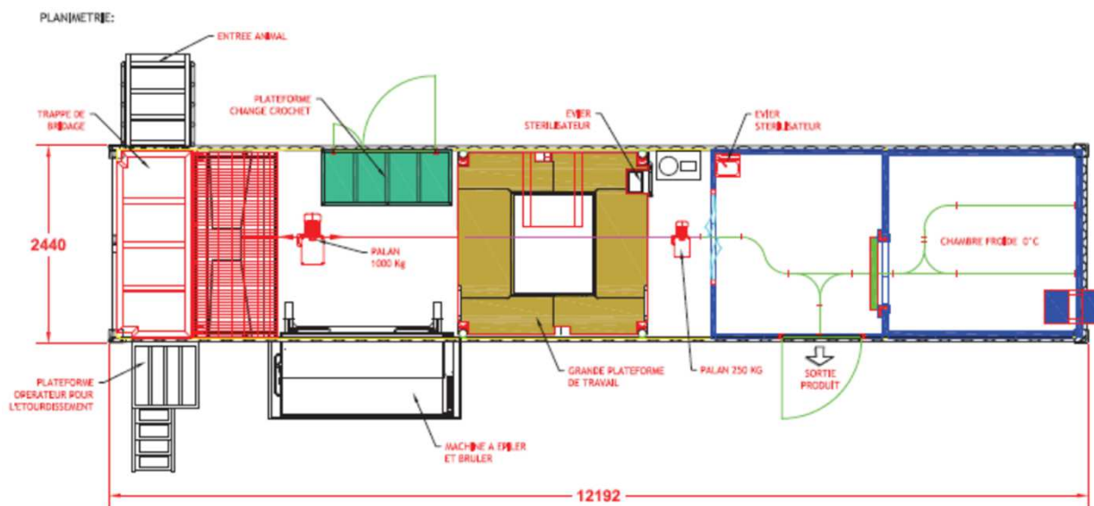
VUE DE DEVANT SCALE 1:200
