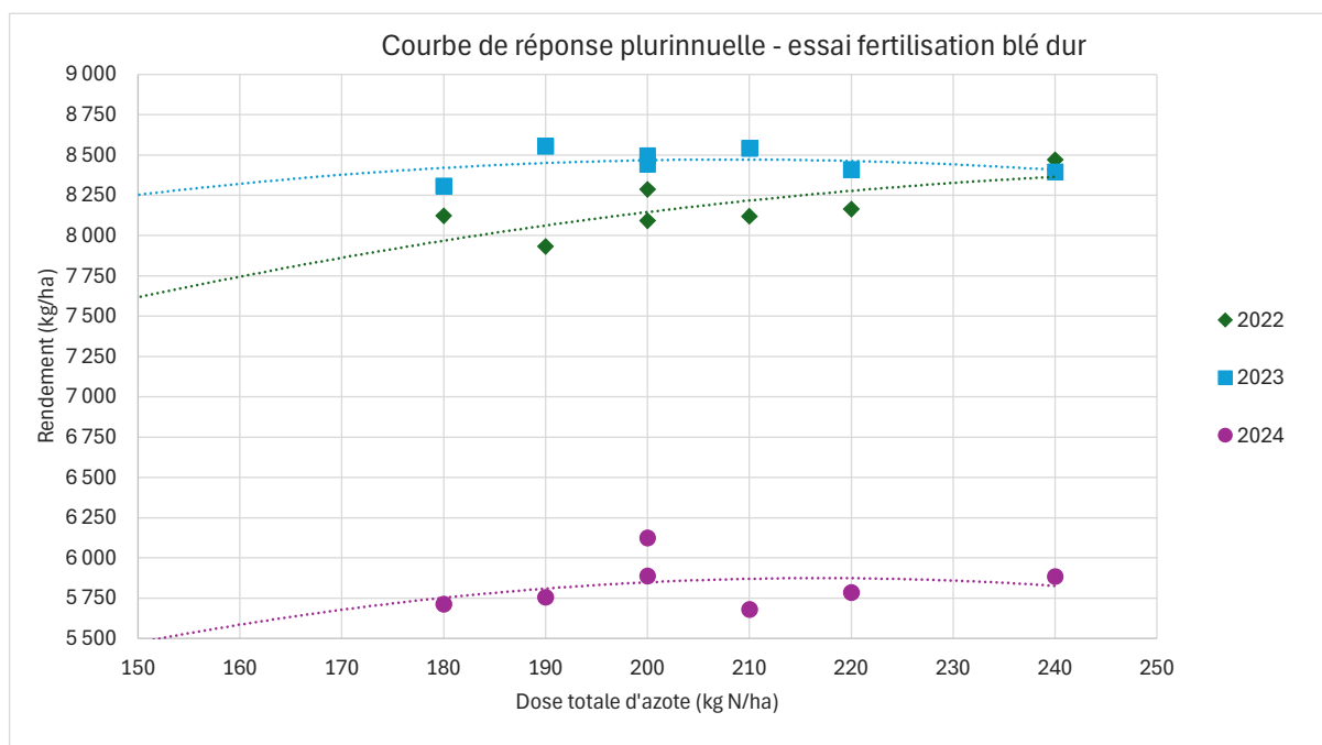
Figure 1 – Courbe de réponse à l'azote dans les essais sur la fertilisation azotée du blé dur menés de 2022 à 2024. Rendement (kg/ha) en fonction de la dose totale d'engrais appliquée (kg N/ha).
